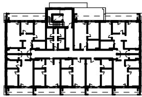
NADSTROPJE
