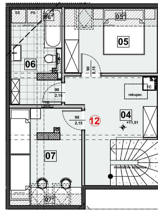
2 MANSARDA 2 1:100
