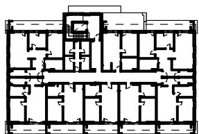
NADSTROPJE
