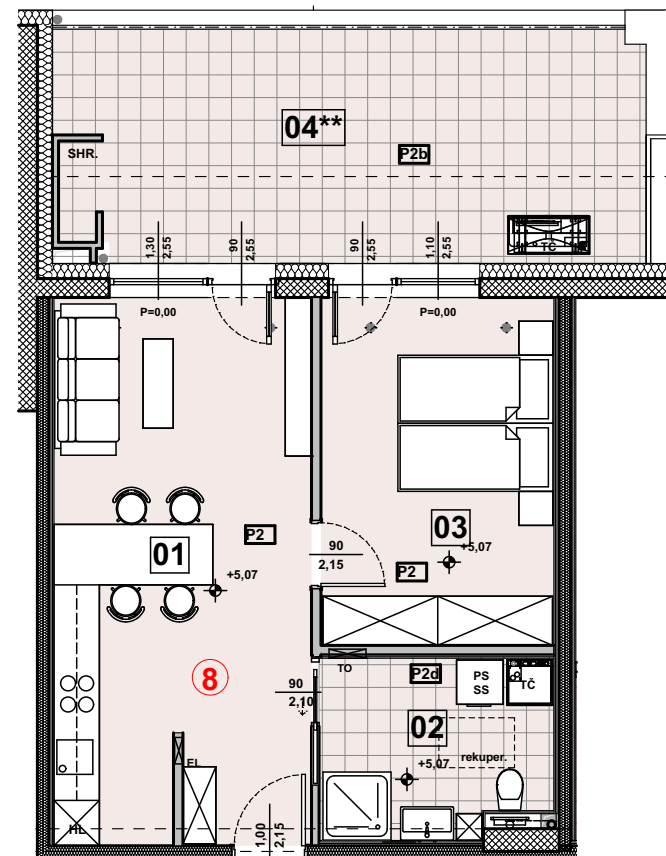
NADSTROPJE
