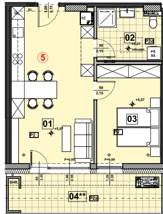
NADSTROPJE
