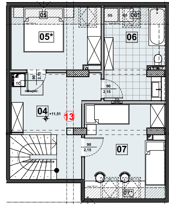
2 MANSARDA 2 1:100
