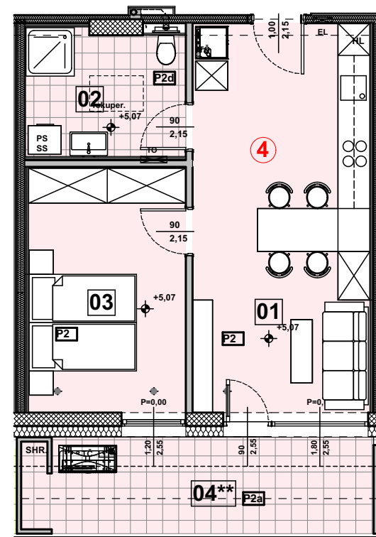
NADSTROPJE
