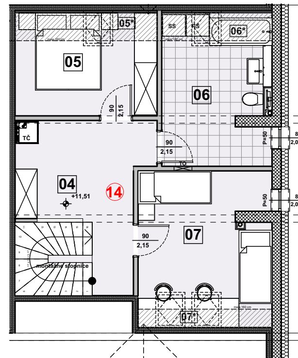
2 MANSARDA 2 1:100
