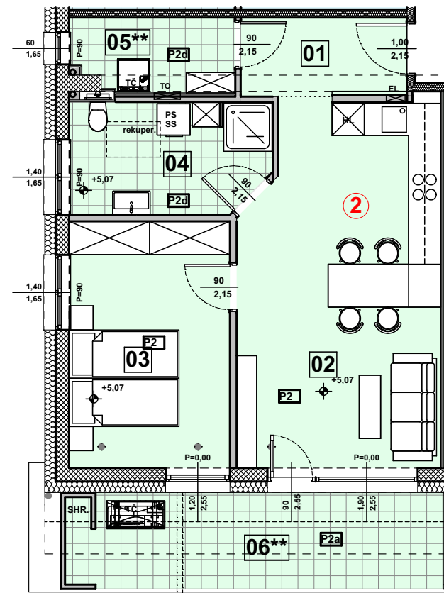
NADSTROPJE
