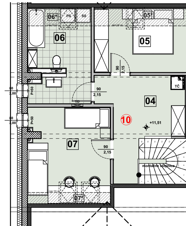
2 MANSARDA 2 1:100
