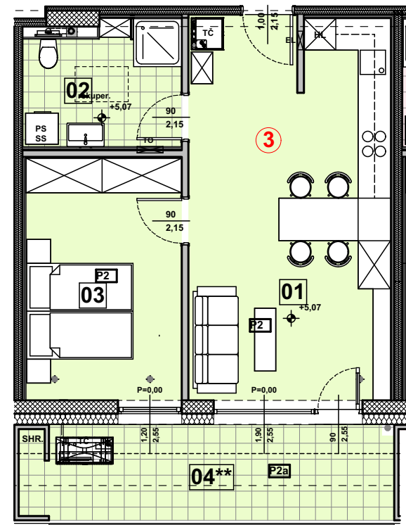
NADSTROPJE
